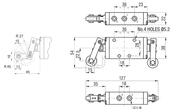
EKCA8/LRLR*
