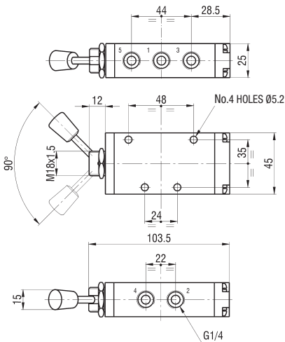
EKCA4/MV - EKCA4/MVF
