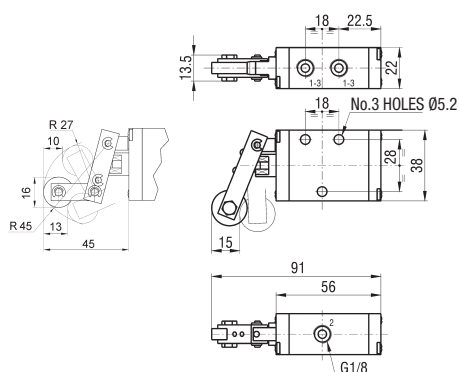
EKCA8/LR*
