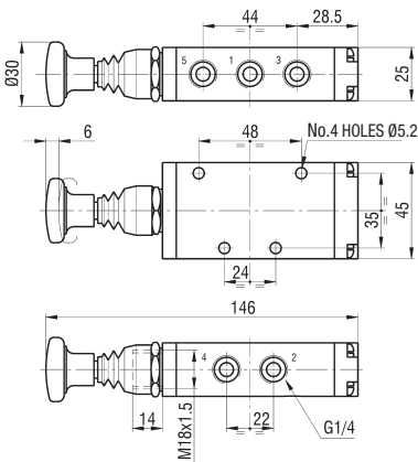
EKCA4/T - EKCA4/TF
