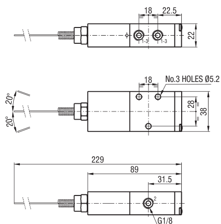
EKA8/A - EKC8/A
