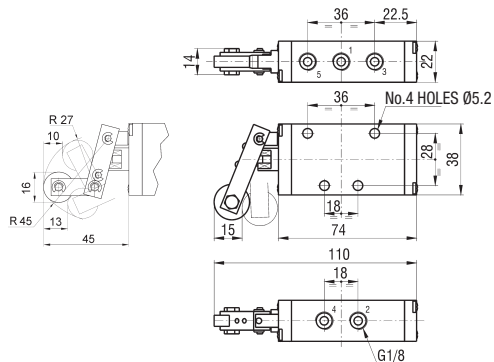
EKCA8/LR*
