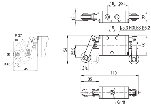
EKCA8/LRLR*
