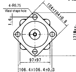
Flange E6
