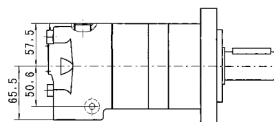
Flange E2
