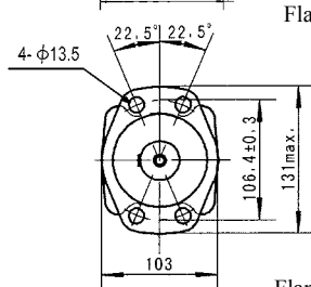
Flange E2B
