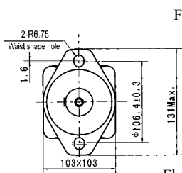
Flange E4
