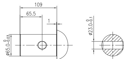
shaft H2
